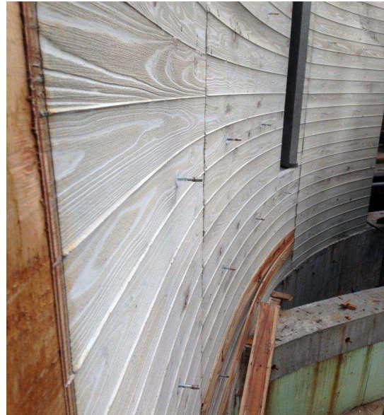
杉板本実実型枠(円形仕上り)
