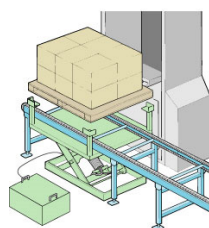
スタッククレーンの受渡し
