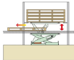
コンベヤライン内90度方向転換
