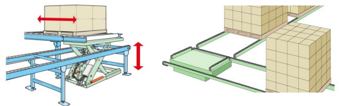
コンベヤライン内90度方向転換
