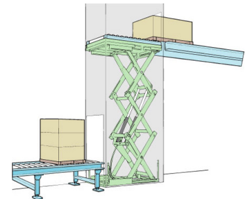
コンベヤライン内90度方向転換
