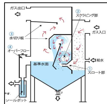
▲ウェットスクラバー
