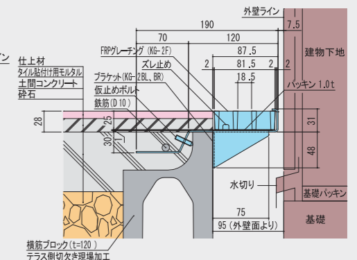
断面詳細図
