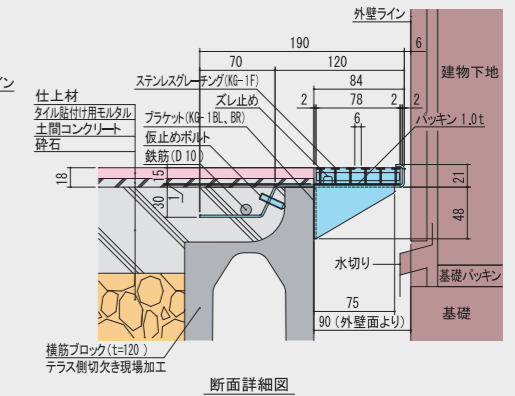
断面詳細図
