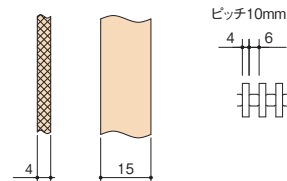
ベアリングバー詳細図
